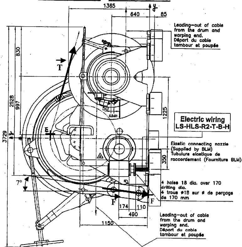
View as per F - Vue suivant F
