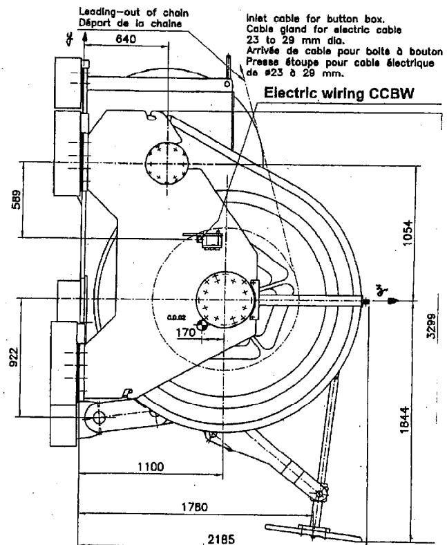
View as per G - Vue suivant G
