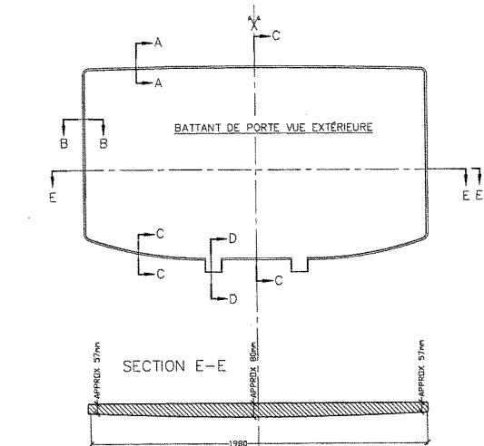
BATTANT DE PORTE Échelle: 1/10
