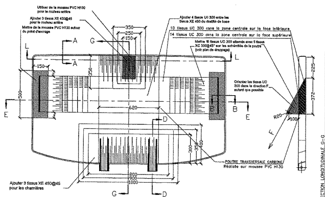
STRUCTURE PORTE COMPOSITE Échelle: 1/10
