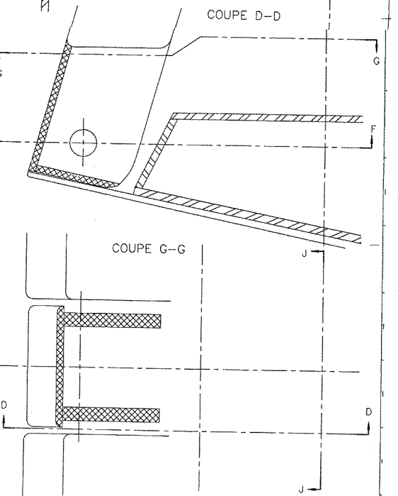
DÉTAIL CHARNIÈRE Éch: 1/1
