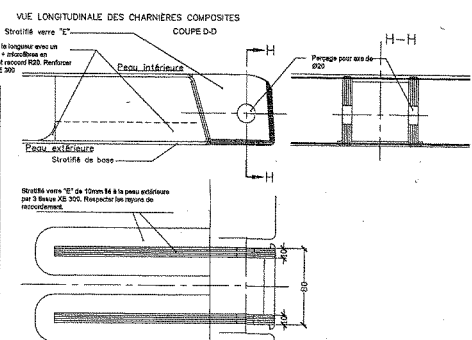
Échelle: 1/2
