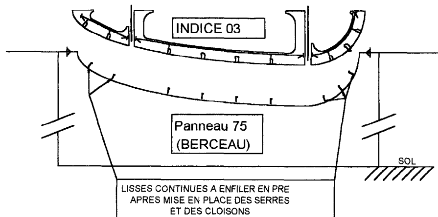
ASSEMBLAGE INDICE 03
