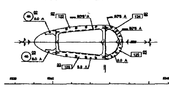
COUPE A 63020/0H
