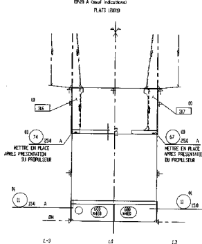
VUE TRANSVERSALE AU C.17-266
