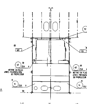
VUE TRANSVERSALE AU C.18+233
