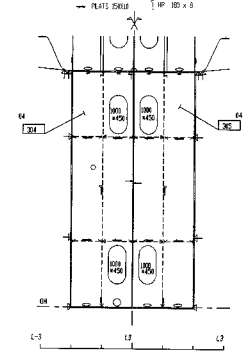
VUE TRANSVERSALE AU C.9
