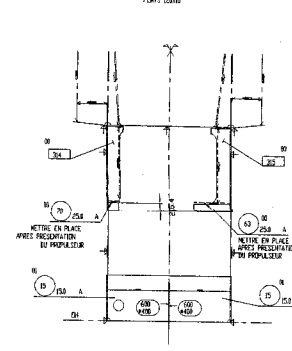
VUE TRANSVERSALE AU C.16-33
